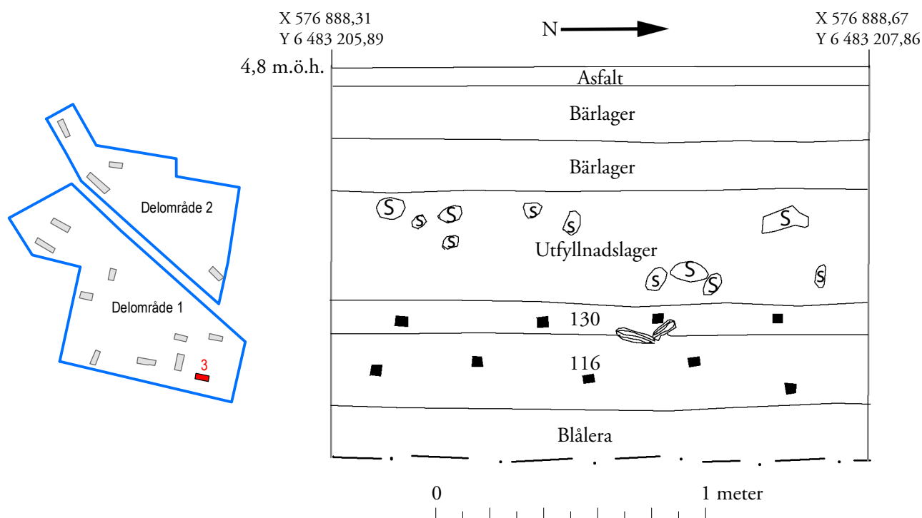
Figur 31. Sektion i schakt 3. Sektionens läge markerat i figur 15.
