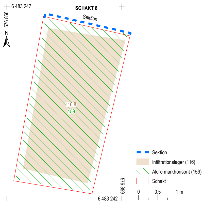
Figur 29. Schakt 8, skala 1:50.
