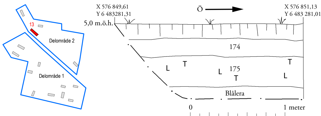
Figur 41. Sektion i schakt 13. Sektionens läge markerat i figur 40.
