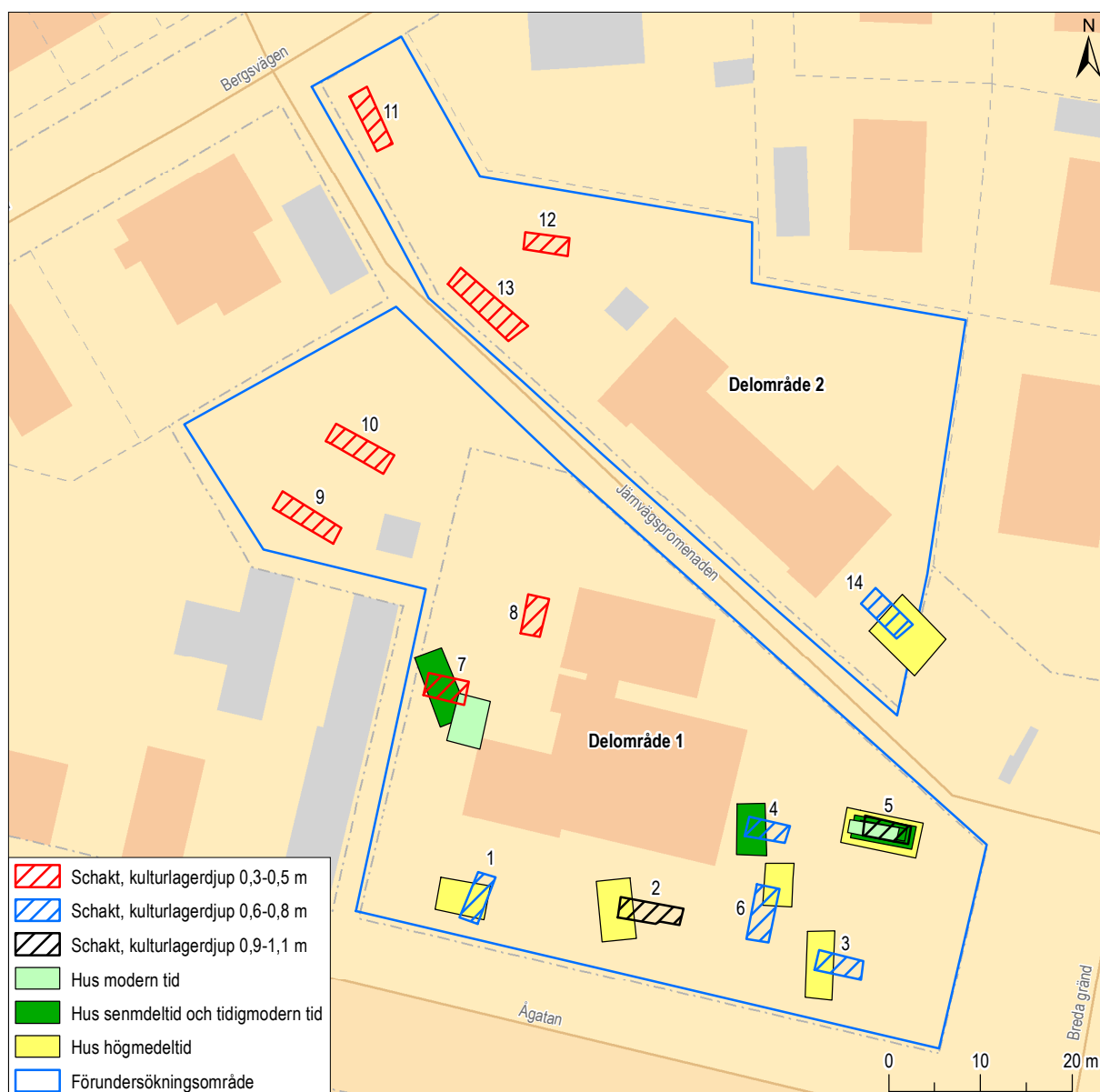
Figur 47. Undersökningsområdet med kulturlagerdjup för respektive schakt samt påträffade hus (eller bebyggelsesår) schablonmässigt markerat. Mot bakgrund av Fastighetskartan, skala 1:750.
